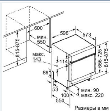
Размерные чертежи
